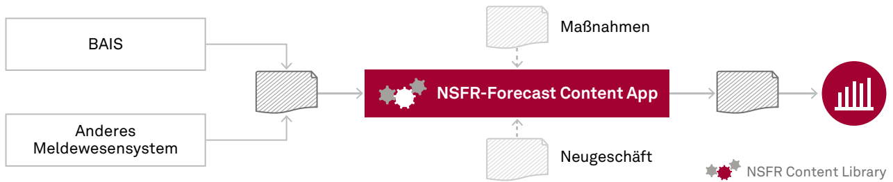
Schematische Darstellung des Zusammenspiels von Meldewesen, NSFR-Forecast Content App und zugelieferter Szenarien
